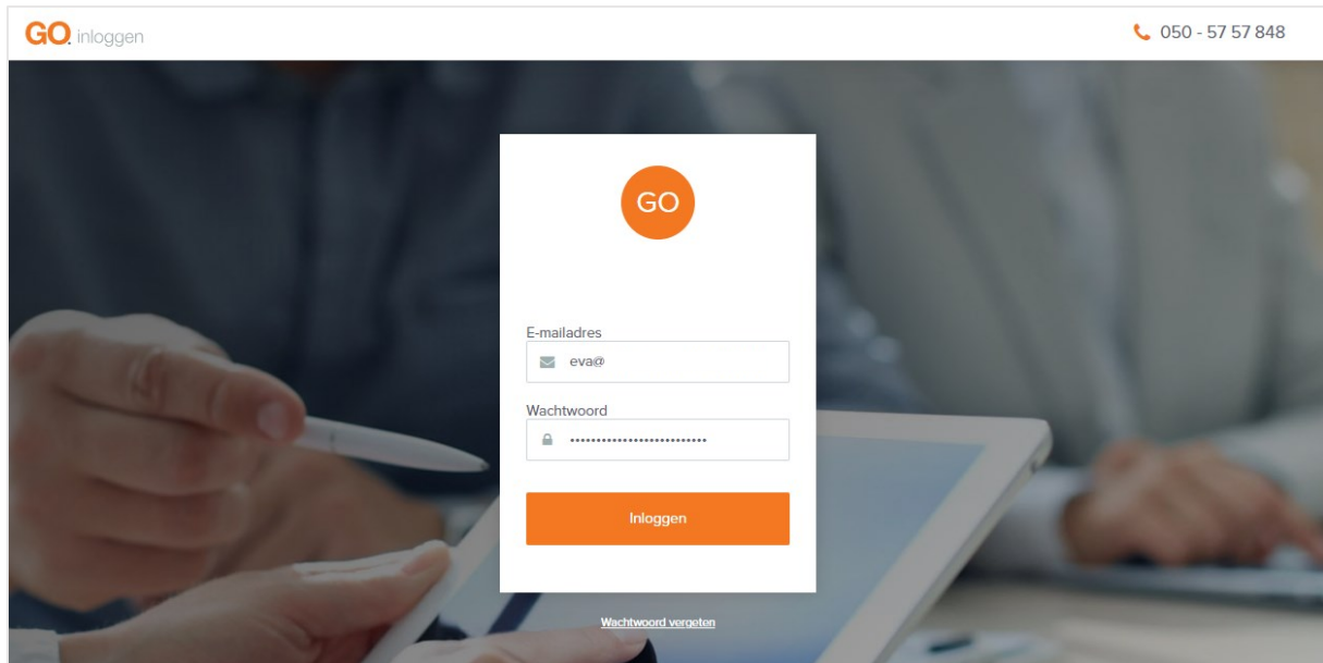
Afbeelding 4 - Inlogscherm
