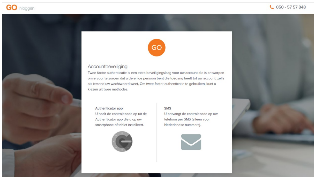
Afbeelding 1 - Instellen 2FA
