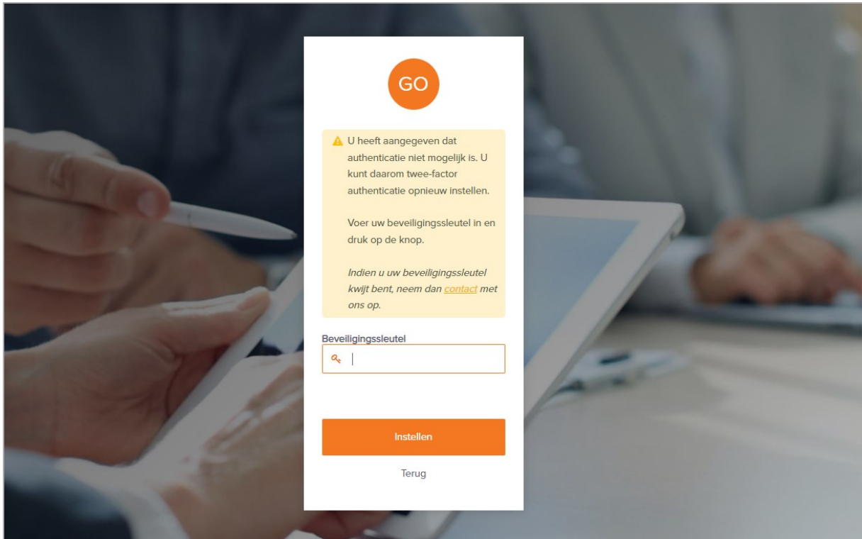
Afbeelding 7 - Beveiligingssleutel invoeren
