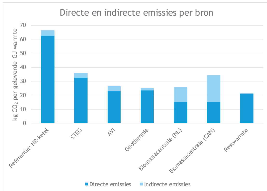
Figuur 9 - Overzicht van ketenemissies per warmtebron
