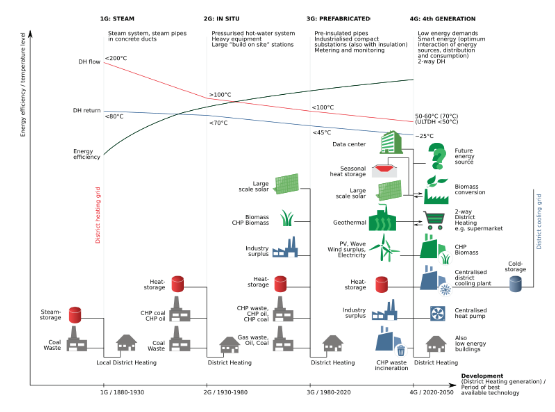
Figuur 2 - Overzicht van generaties van warmtenetten
