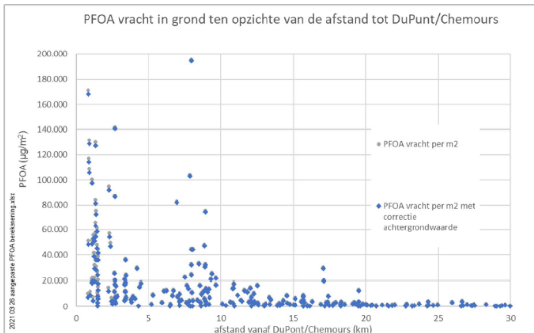
Figuur 10 Uitgerekende PFOA-vracht in de bovenste 2 meter van de bodem, geplot ten opzichte van de afstand vanaf het terrein van DuPont/Chemours voor alle windrichtingen. Waarden waarvan het droge stofgehaltes niet bekend, zijn niet omgerekend, vandaar dat er minder punten zijn dan in de eerdere figuur met PFOA per \mu\text{g}/\text{kg} geplot ten opzichte van de bron. Weergegeven in grijs is de PFOA-vracht berekend zonder correcties, waarden in blauw zijn gecorrigeerd voor de diffuse achtergrondbelasting met PFOA.
